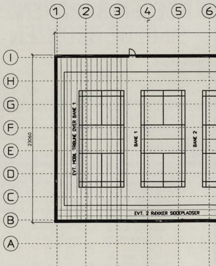
Skitse til det nye halbyggeri, udført af arkitekt og ingeniørfirmaet Wolfsberg & Lindhardt i Skælskør.
