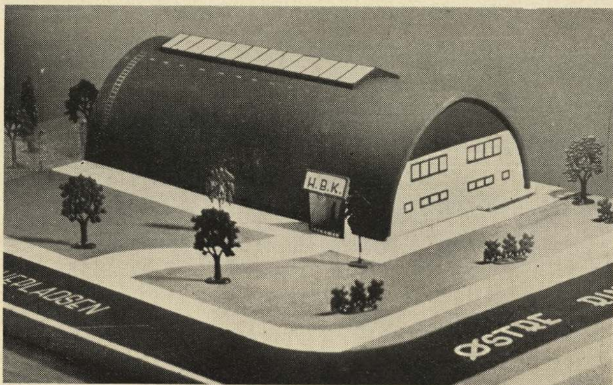
Den projekterede hal i Hjørring. (Fot. Steen Sørensen, cliché: Vendsyssel Tidende).
